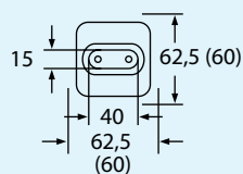
Bild 32: Einbaumaße und Strahlerabmessungen ( ) in mm
